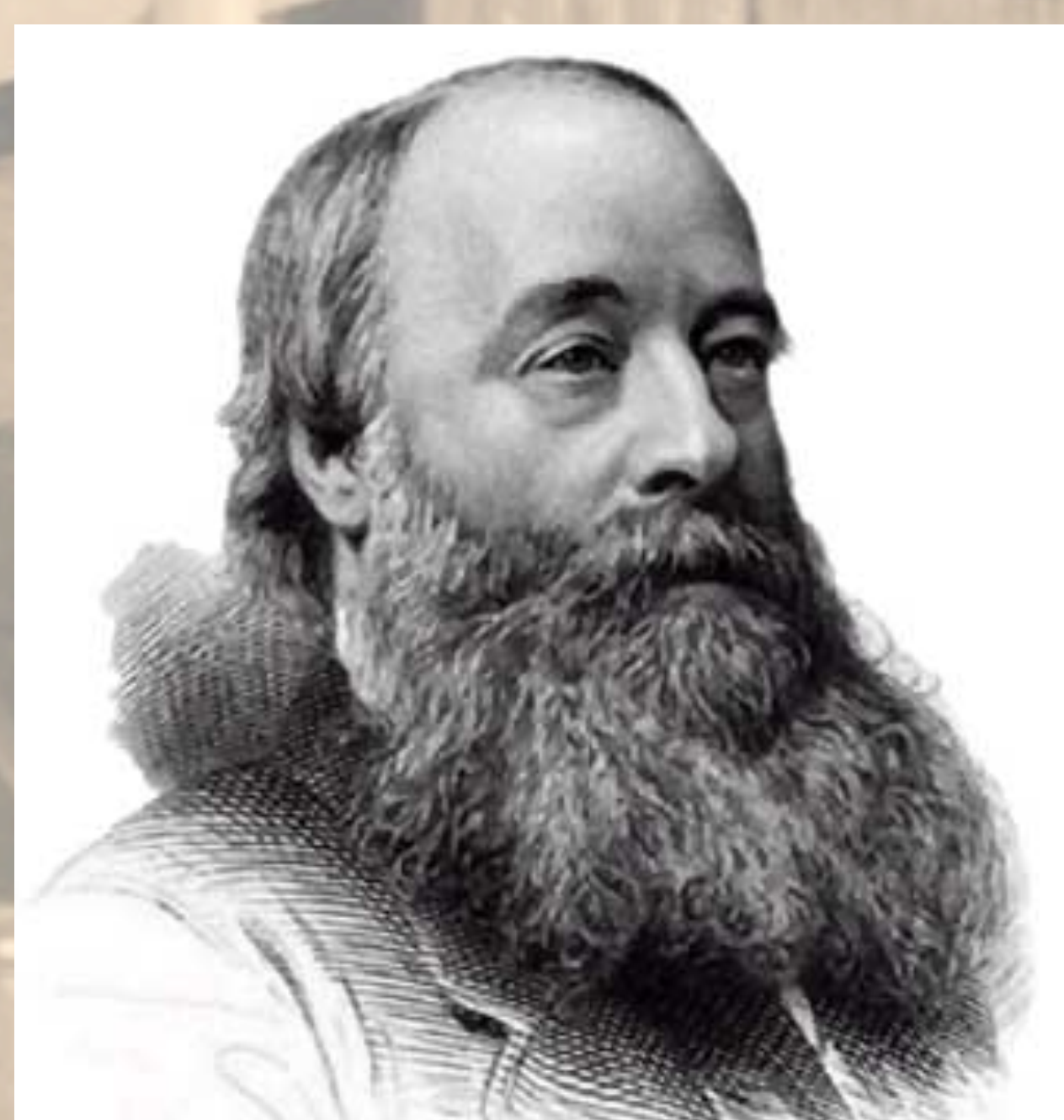
James Joule 1818-1889
