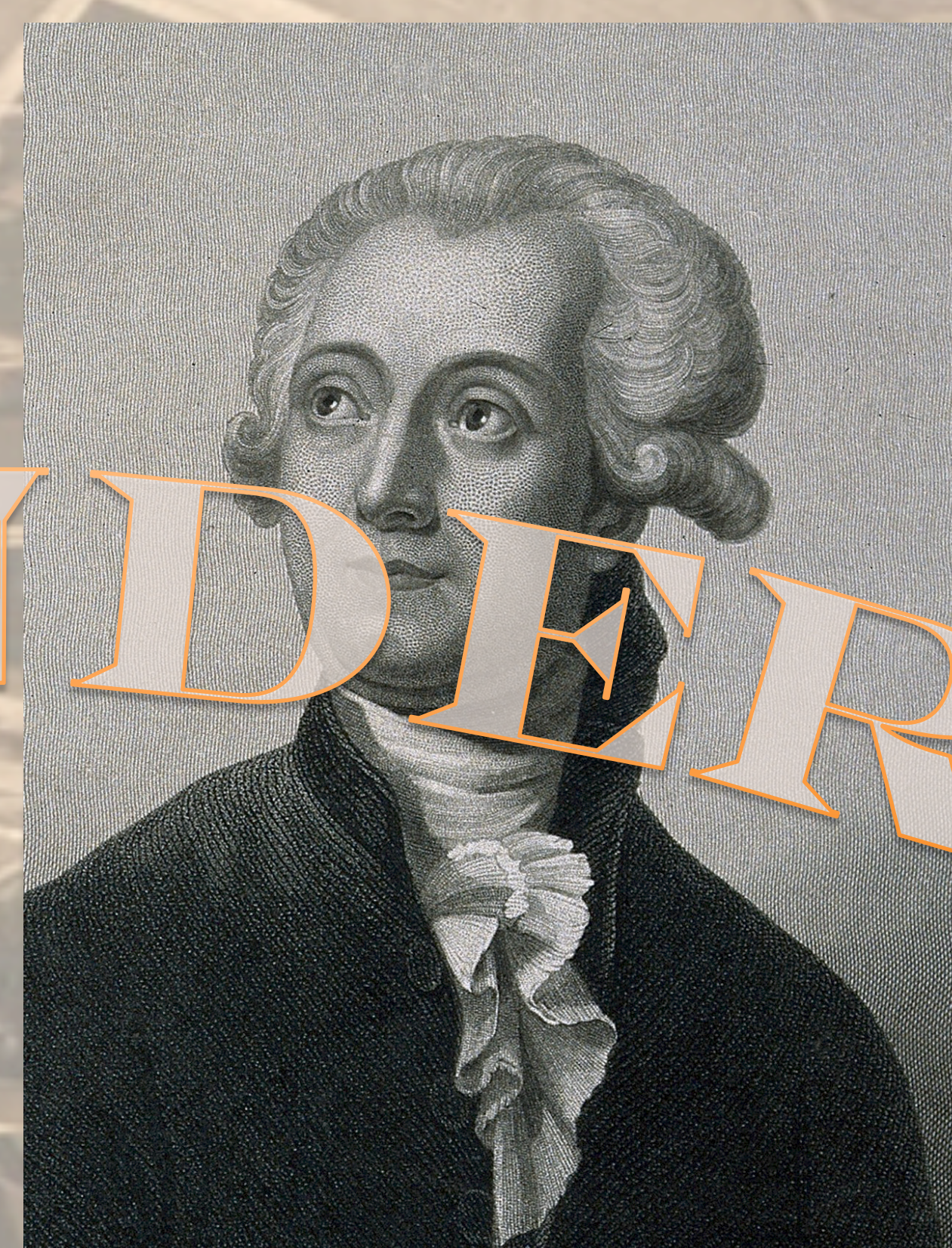
Antoine Lavoisier 1743-1794
