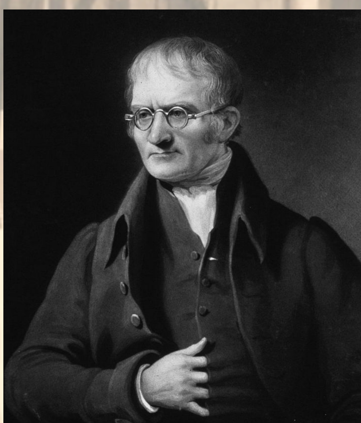
John Dalton 1766-1844
