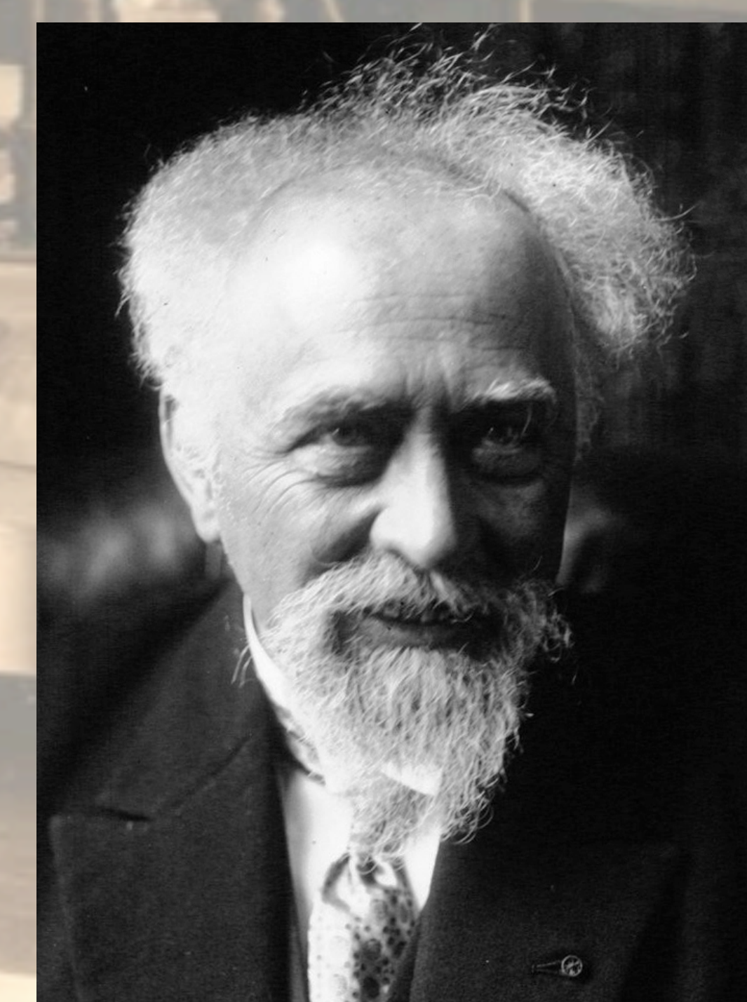
Jean Perrin 1870-1942
