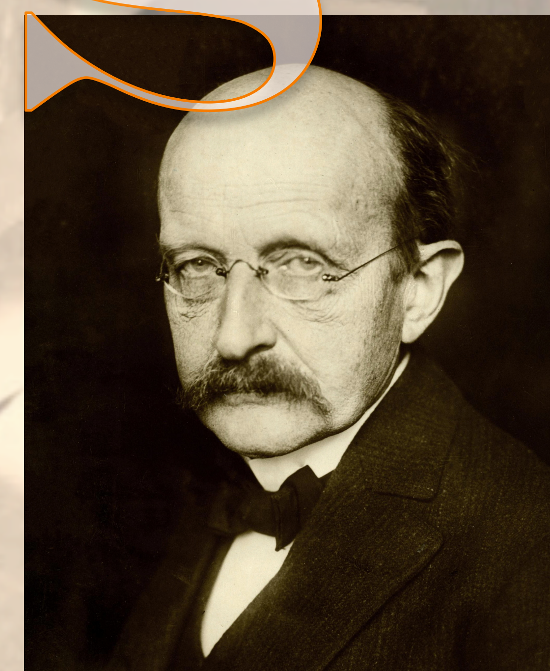
Max Planck 1858-1947
